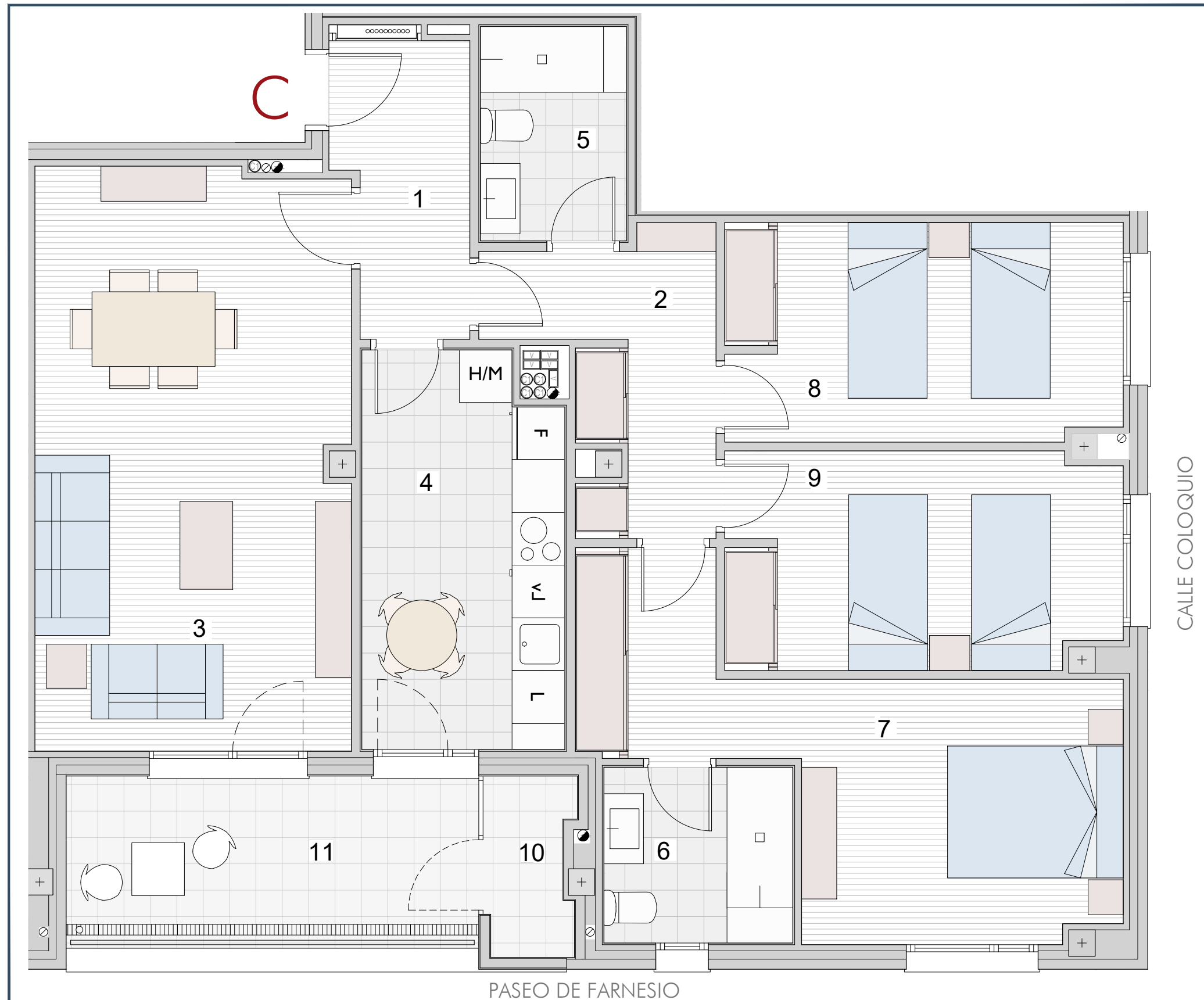
PLANTA 1ª a 4ª
